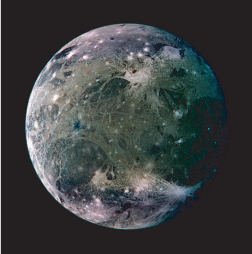
Fig. 2.45 Jupiter's satellite Ganymede
